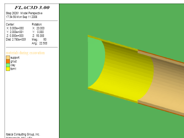
Excavation: tunnelier (jaune), soutènement, et colis (orange)
