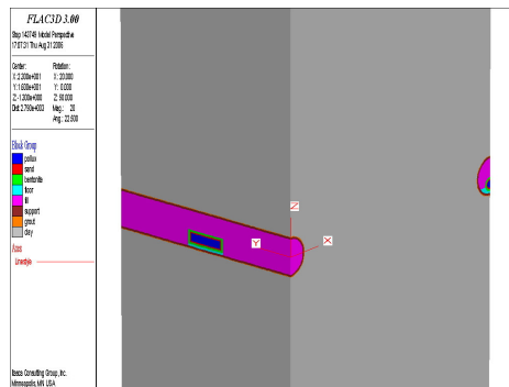
Tunnel (rose) et disposition des colis de stockage (bleu), site Nord
