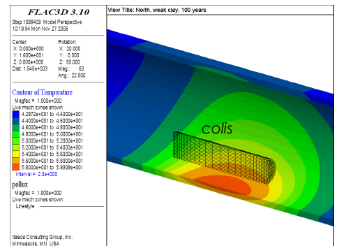
Températures dans le soutènement après 100 ans de chauffage, site Nord
